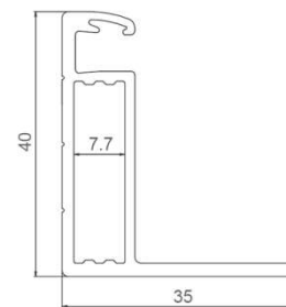
A-A
