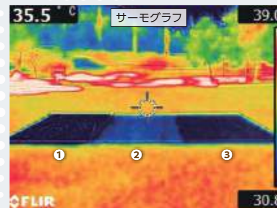
①当社アルミ蒸着タイプ②当社白ネット③バロンスクリーンホワイト涼風(土の温度34.2°C)
