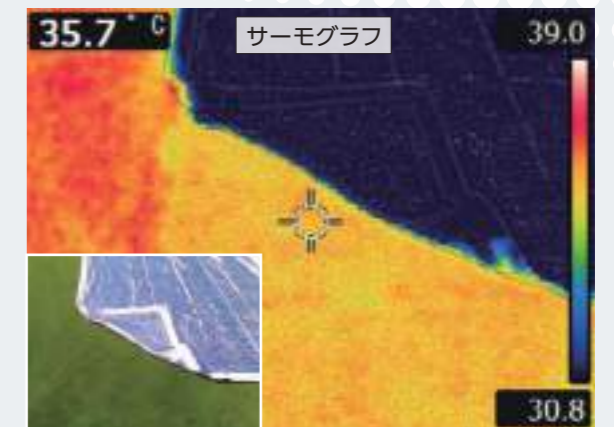
①当社アルミ蒸着タイプ(土の温度35.7°C)
