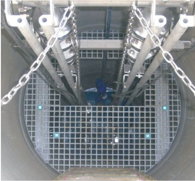
Φ1500用ポンプスラブ
