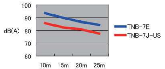
騒音値比較: 標準(7E)対静音(7J-US)
