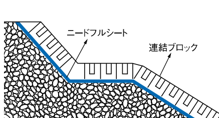
② 吸出防止工法
