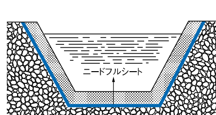
③ 導水路の吸出防止工法
