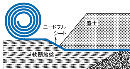
① 軟弱地盤土地改良工法
