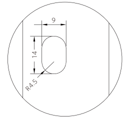
1部取付固定穴拡大図
