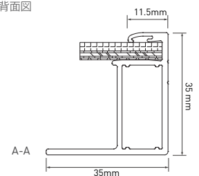
背面図
