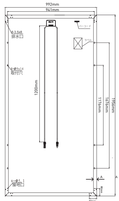
背面図
