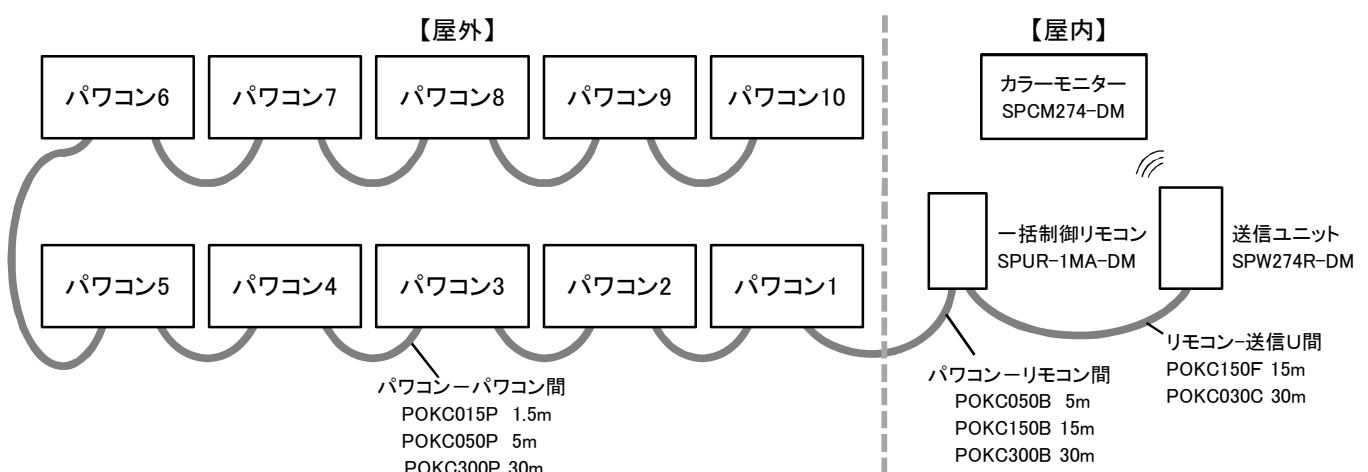
パワーコンディショナとパワーコンディショナDIPスイッチ、リモコンサービススイッチ組み合わせ表
