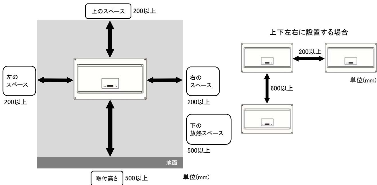
図7-1 壁面取り付け時の周囲との最低スペース
