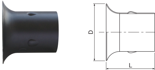
品番: KBM-□□□ (例) φ30の場合 KBM-030
