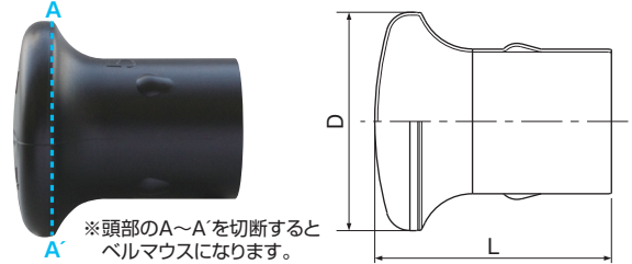
品番: KYB-□□□ (例) φ30の場合 KYB-030
