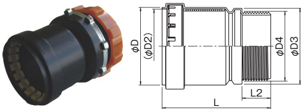
品番: KBS-□□□ (例) φ30の場合 KBS-030
