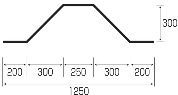
形状および寸法 (mm)
