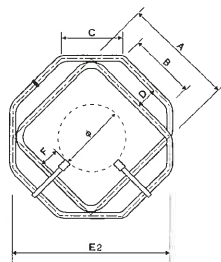
② 1箇所溶接型
