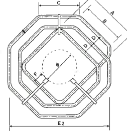
④ 1箇所溶接型3重リング
