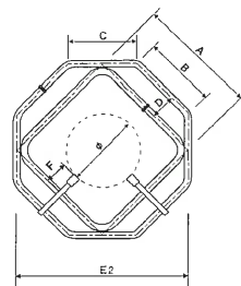
③ 2箇所溶接型
