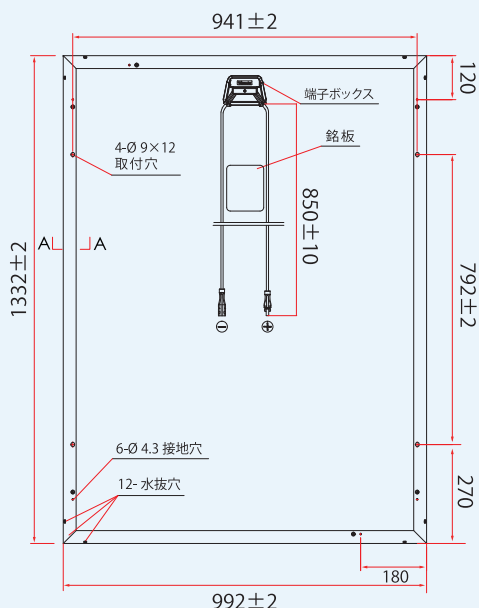
背面図
