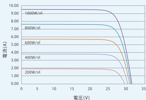
PVモジュール TSM-DC03A.08(II)230Wの I-V 曲線
